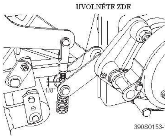
Obr. 6-1 Seřízení brzdy
