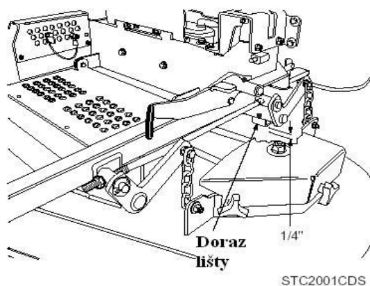
Obr. 6-7 Doraz žacího ústrojí
