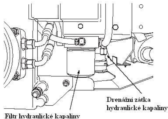
Obr. 7-3 Hydraulický filtr a drenážní zátka
